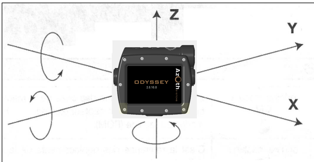
Mouvements de rotation pour calibrer la boussole numérique
